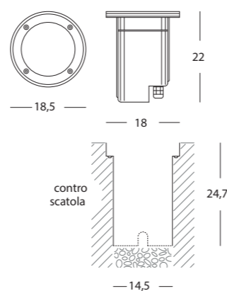
art. 227/09 acciaio Lampada H max 145 mm EAN: 8020588850004 con parabola riflettente in alluminio
